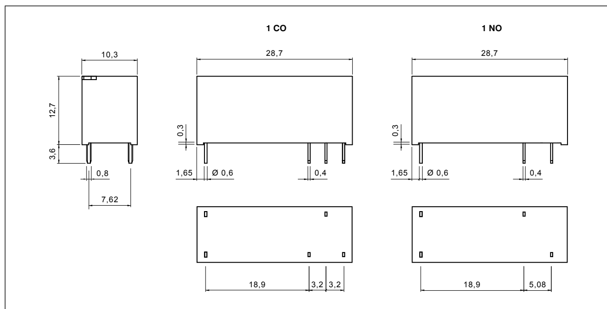
Габаритные размеры
