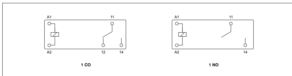
Схемы коммутации (вид со стороны выводов)
