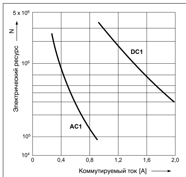
Электрический ресурс по функции тока нагрузки. Частота коммутации: 1 800 циклов/час
