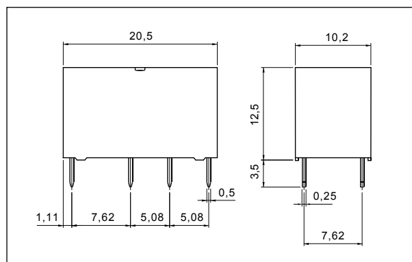
Габаритные размеры
