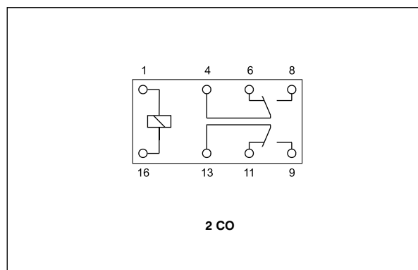
Схема коммутации (вид со стороны выводов)
